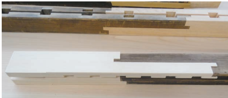
図2 継木された古材
