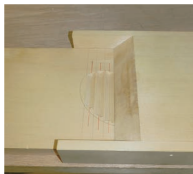
図9 棧唐戸下面の格狭間文様加工中 （正確な作業を行うための道具も作る）
