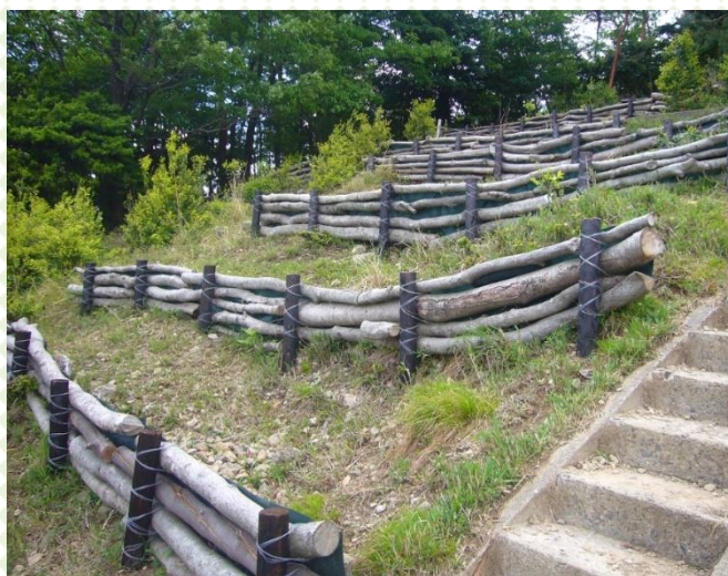
土留めシガラ柵を設置する
